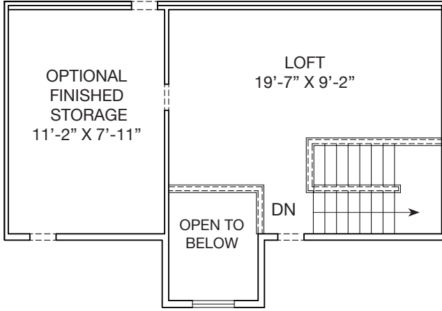
OPTIONAL LOFT
