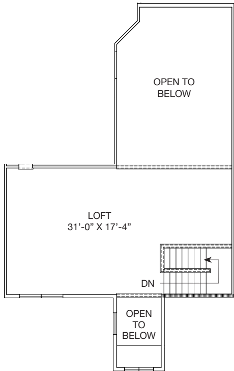
OPTIONAL LOFT
